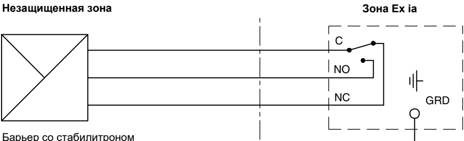
Барьер со стабилизатором Коммутирующий усилитель NAMUR
