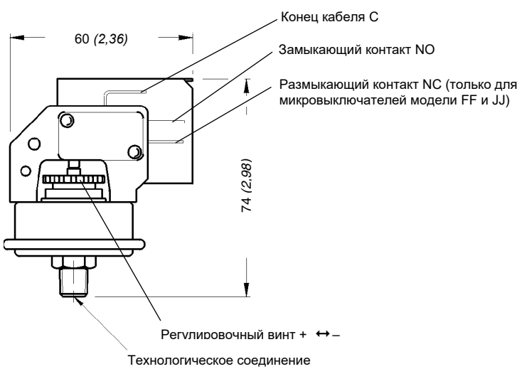
Рис. 11: Мембранно-поршневое реле давления модели MSPS-...
