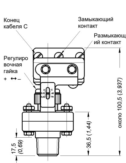
Рис. 7: Мембранно-поршневое реле давления модели E1S-...
