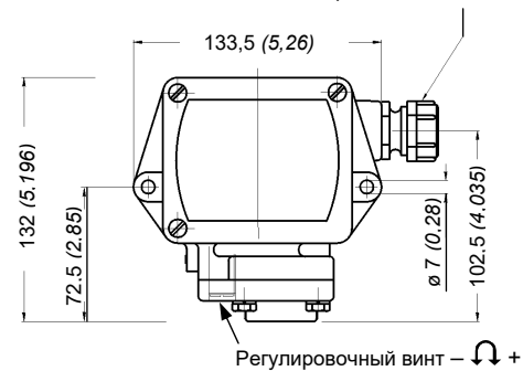
Рис. 9: Мембранно-поршневое реле давления модели P1H-...
