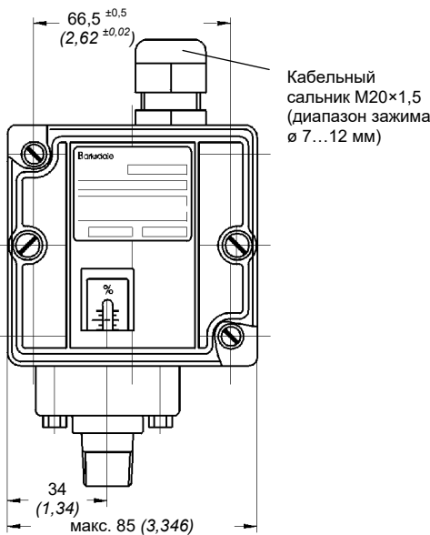
Рис. 8: Мембранно-поршневое реле давления модели E1H-...
