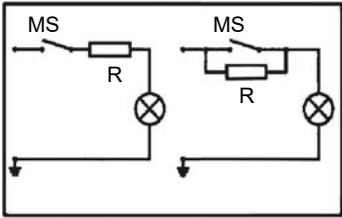
Рис. 2: Ламповая нагрузка и параллельным или последовательным сопротивлением относительно реле
