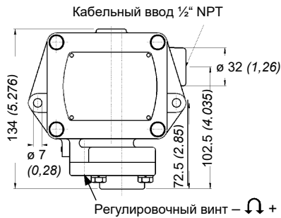
Рис. 10: Мембранно-поршневое реле давления модели P1X-...
