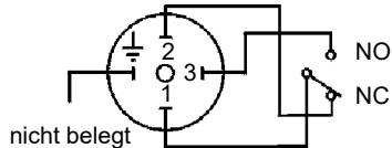
Bild 5: Schalt- und Anschlusschema
