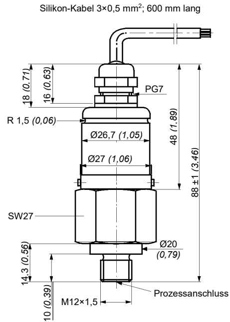
Bild 7: Kolben-Druckschalter Typ KD1-...-K2
