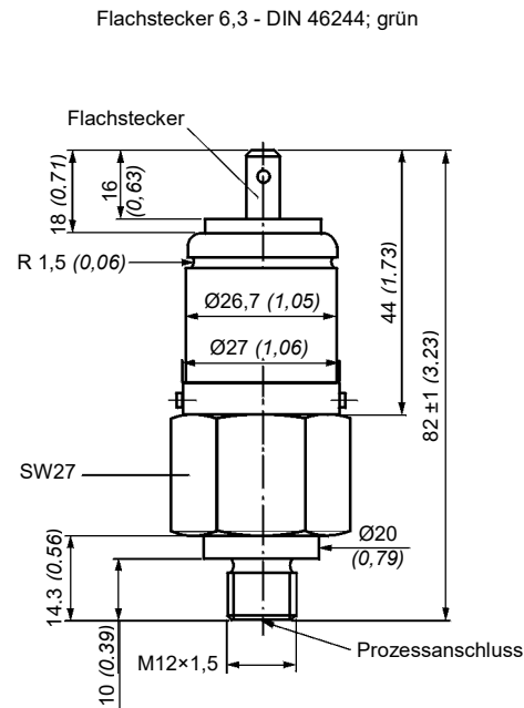
Bild 8: Kolben-Druckschalter Typ KD1-...-A1
