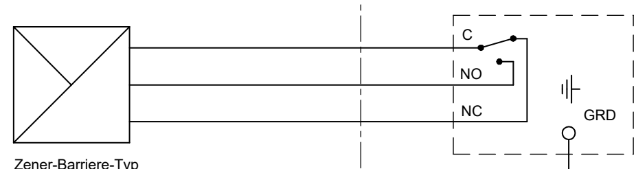
Bild 6: Betreiben von Druckschaltern in eigensicheren Bereichen
